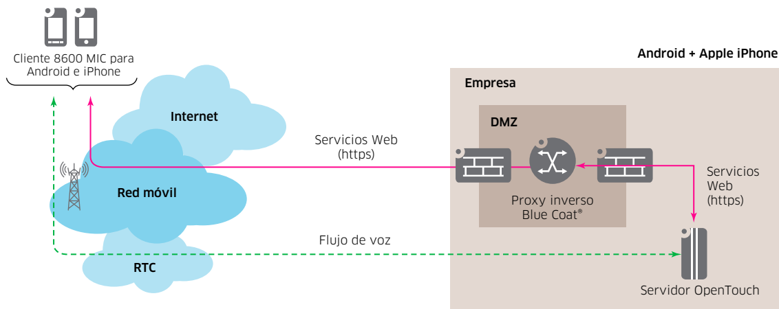
Figura 1. Protección de las conversaciones móviles: ejemplo de arquitectura de red
